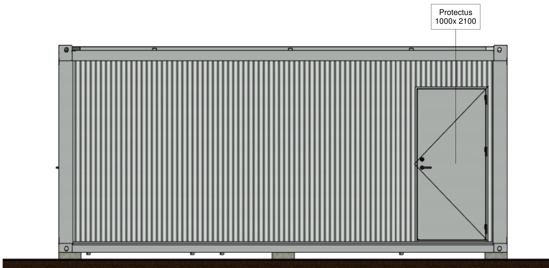
3 Vakarinis Fasadas 1 : 25
