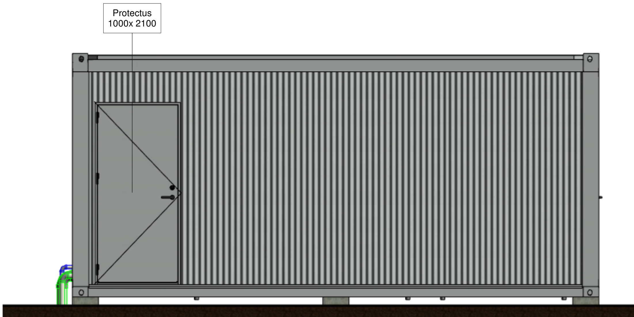
3 Vakarinis Fasadas 1 : 25
